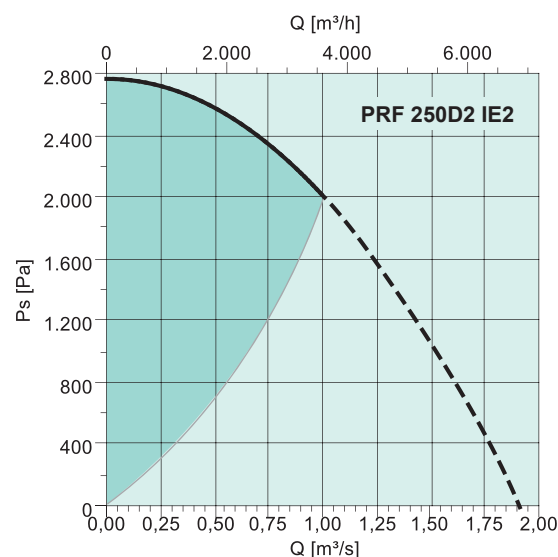
минимальное обратное давление, 2000 Па
