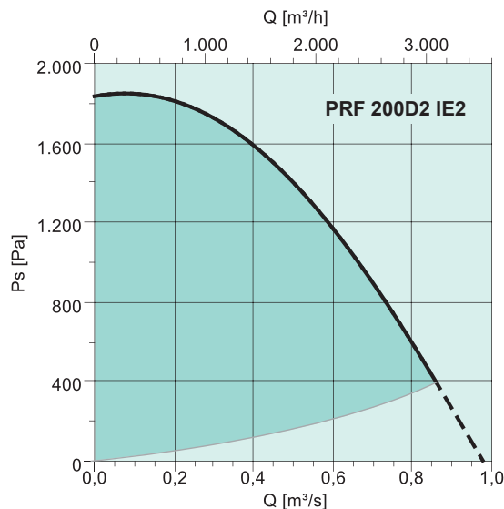
минимальное обратное давление, 400 Па
