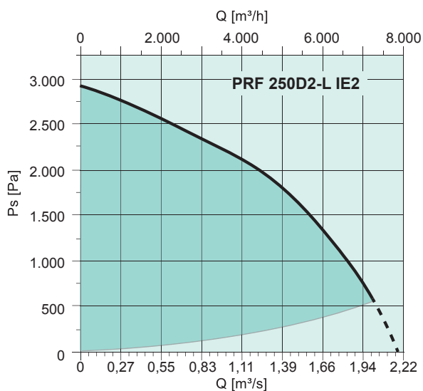
минимальное обратное давление, 550 Па
